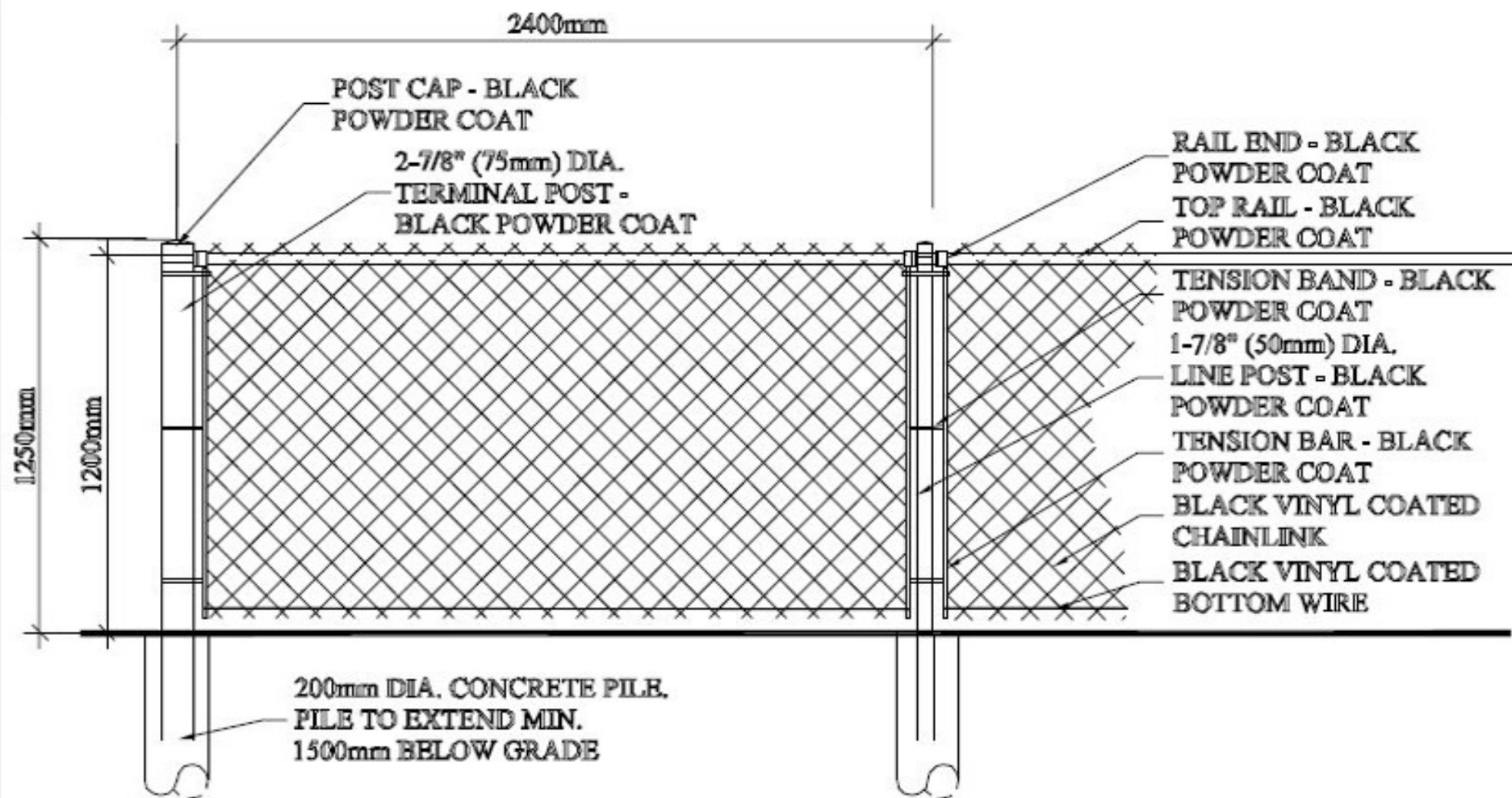
ELEVATION
