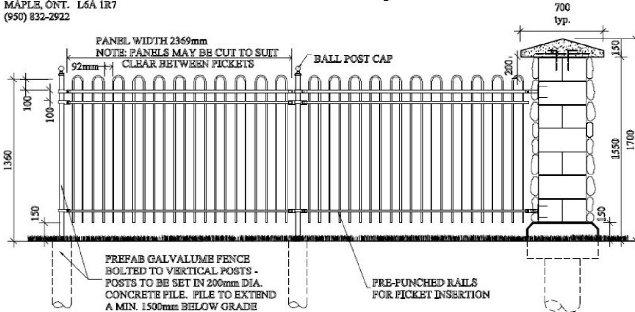
ELEVATION
